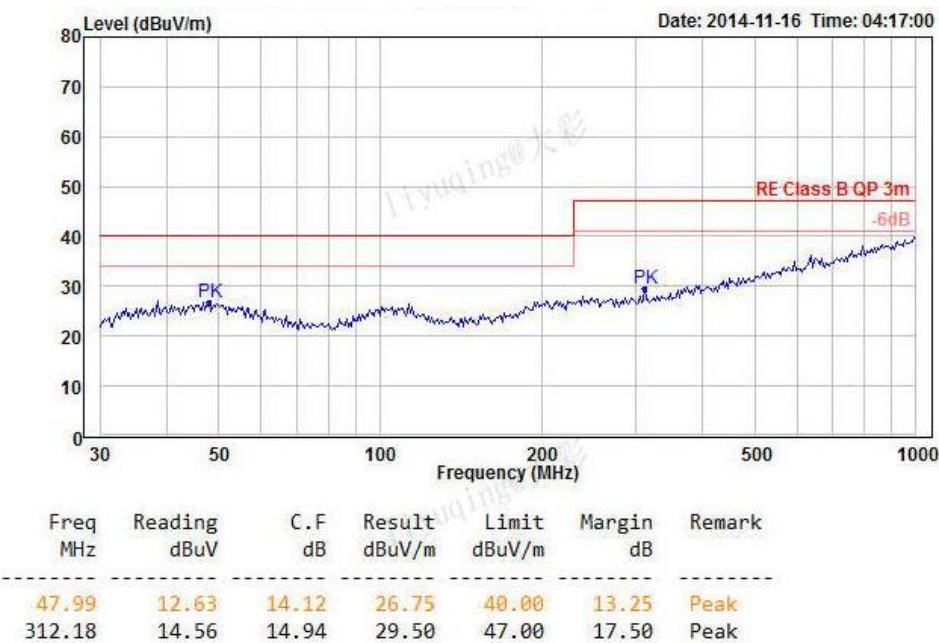
图 5-8 辐射测试垂直方向
