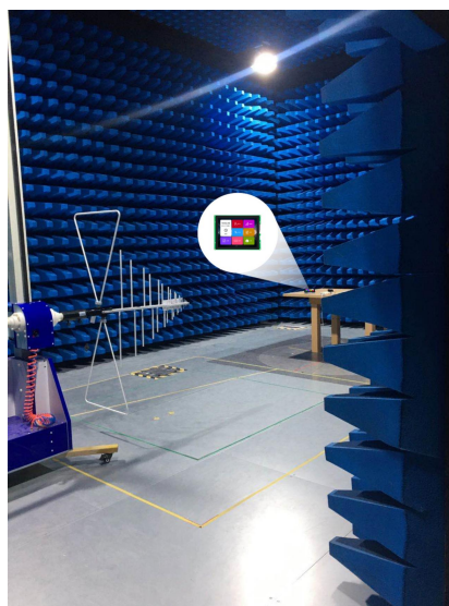
图 5-6 辐射测试图
