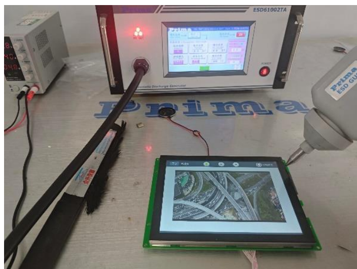
图 5-2 ESD 测试图
