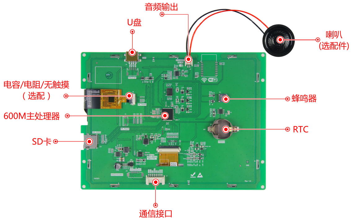
图 1-4 硬件配置图
