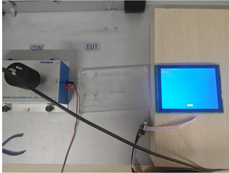
图 5-5 传导抗扰度测试图
