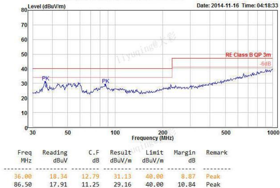
图 5-7 辐射测试水平方向
